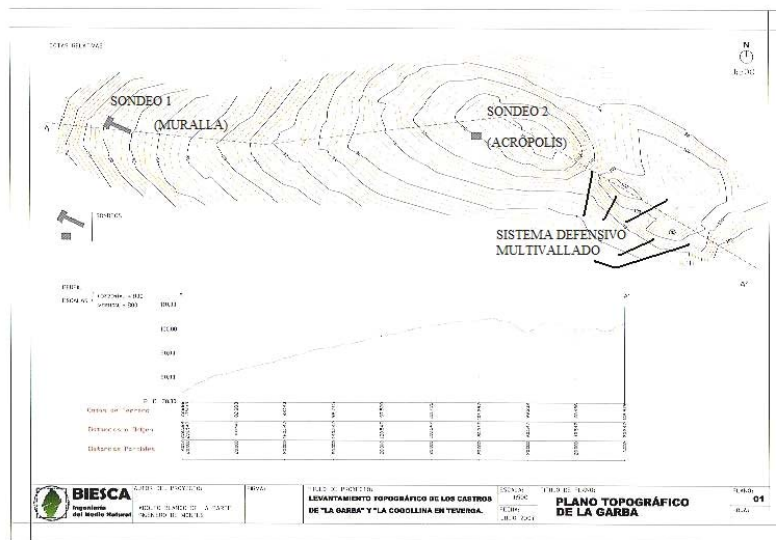
Figura 2. Topografía del castro de la Garba, con la señalización de los sondeos realizados y de la morfología del poblado.
