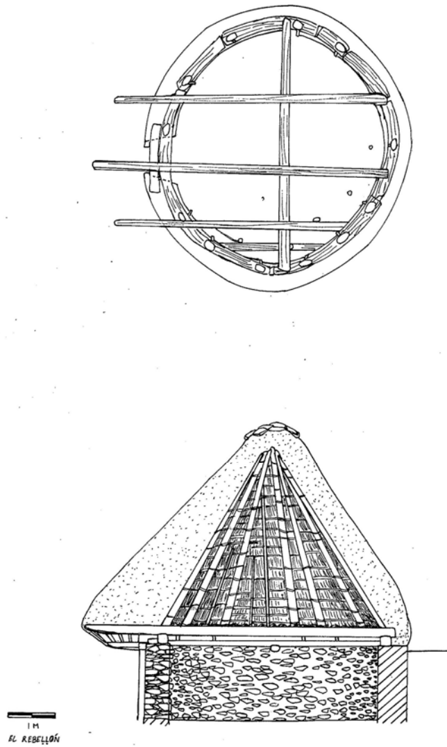
Figura 6. Planta y perfil de la estructura ganadera circular del Rebel.lón / Rebechón.
