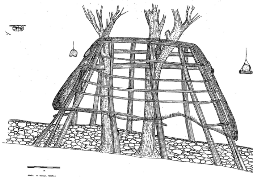
Figura 5. Perfil de la estructura de hábitat puntual del Troncu, en Teverga.
